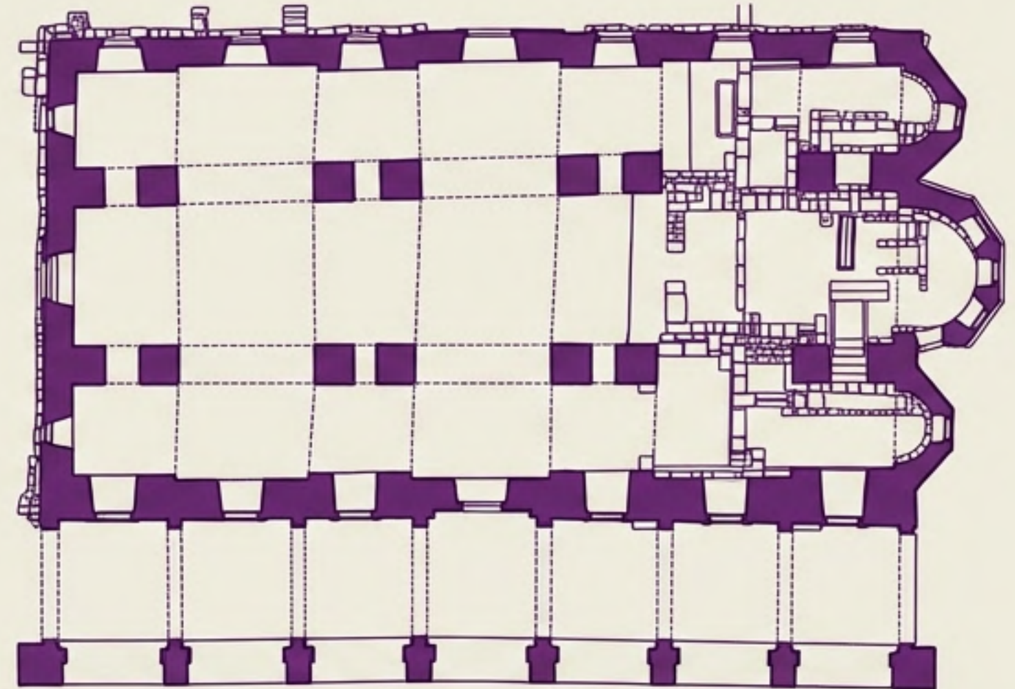
ΚΑΤΟΨΗ
